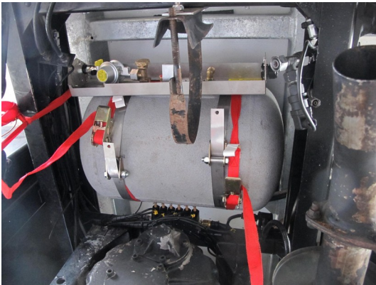
Gastank, unterflur
